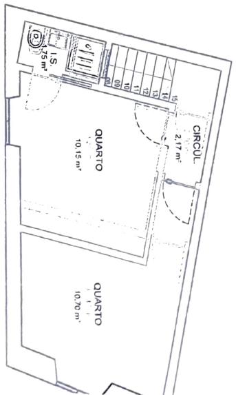
PISO 2
