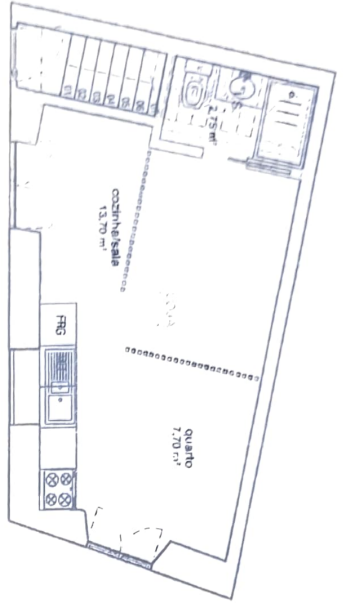
PISO 0
